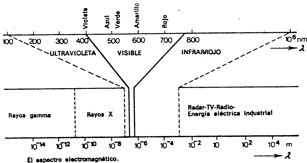
Fig. El Espectro Electromagnético. Se observa el reducido rango dentro del cual los seres humanos pueden percibir visualmente lo que los rodea.
